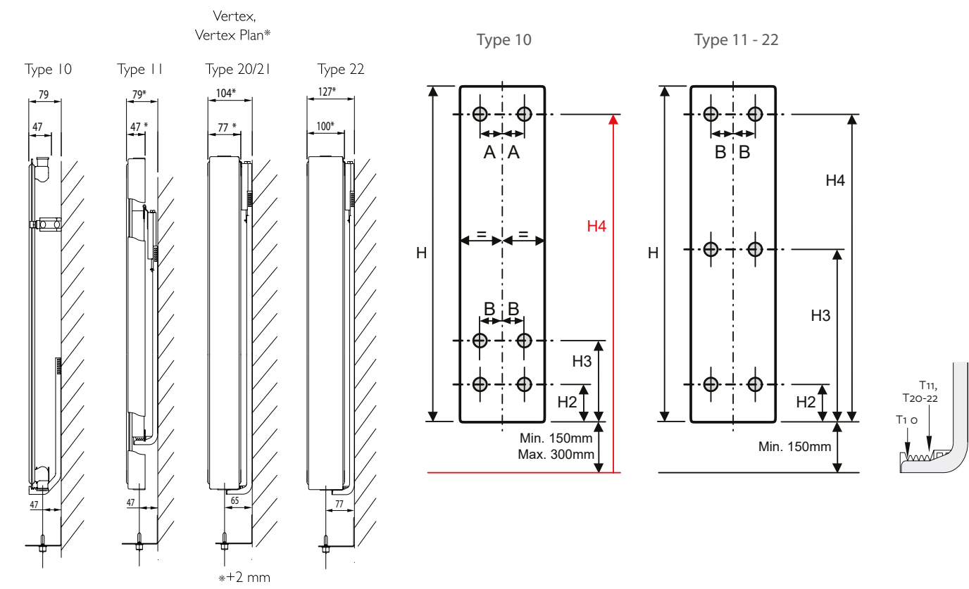
Borehullernes placering på beslagene
