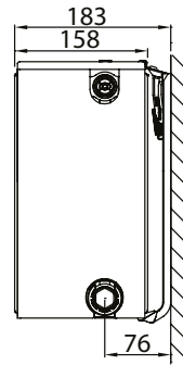
Type 33
