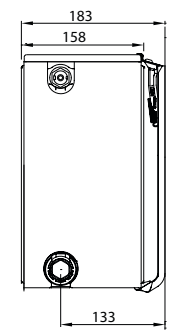
Type 33 Venstre
