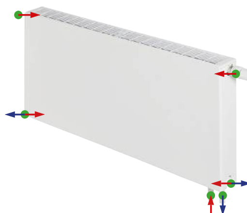
PLAN 6 RADIATOR MED 6 ANBORINGER
