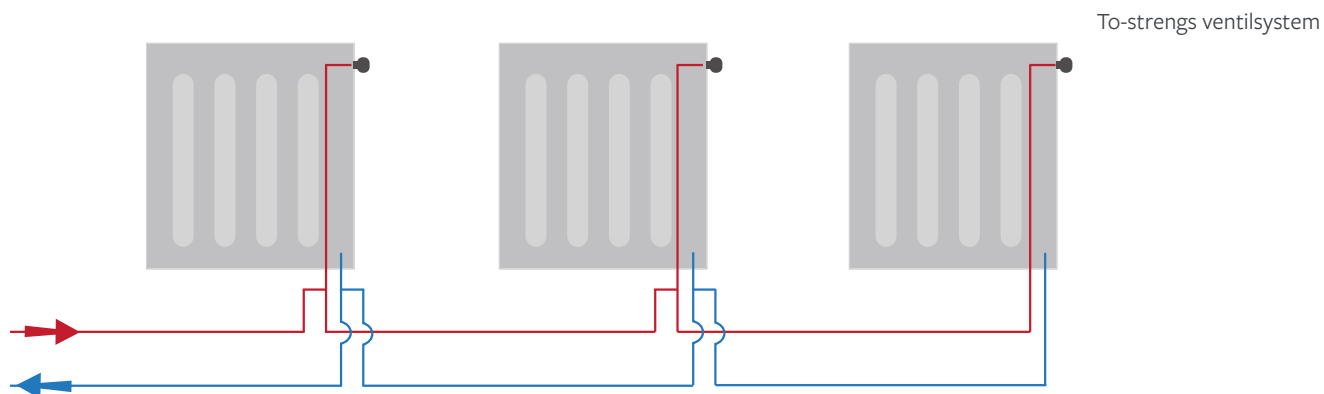
To-strengs ventilsystem med omvendt retur
